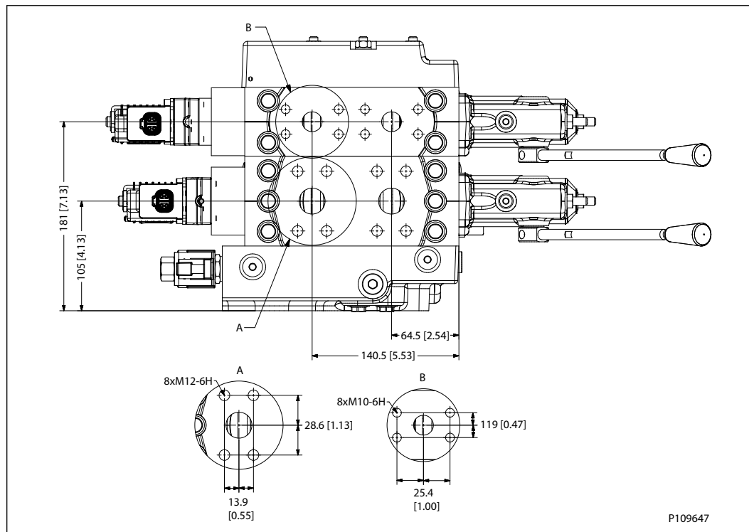
PVG 128/256 尺寸
