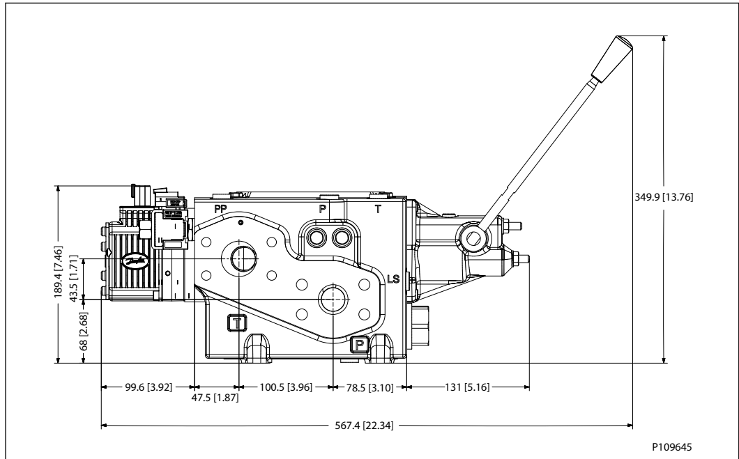
PVEH
