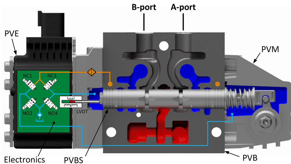
PVG 32 带 PVEH/PVES
