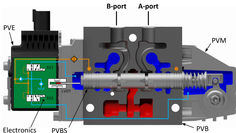
PVG 32 带 PVEO/PVEM (PVEO 不带 LVDT)
